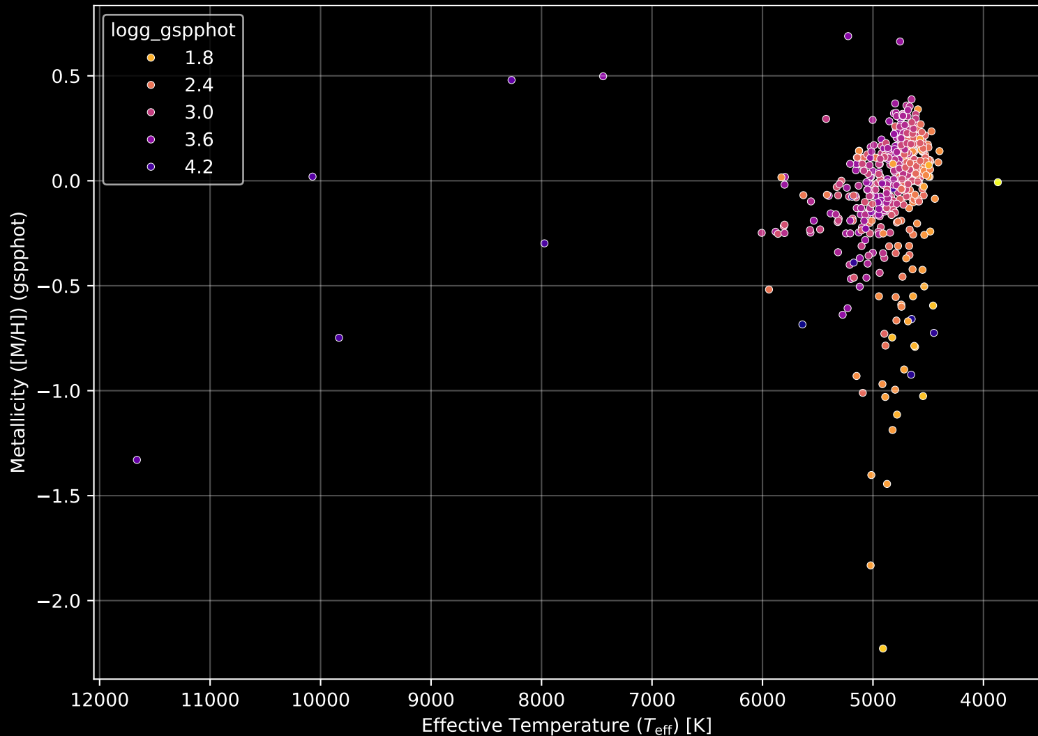
APOGEE DR17 Field: [340-06] Stellar Population Parameters (n= 464)
